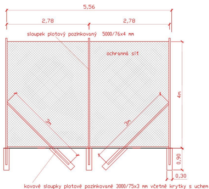
VÝŘEZ OPLOCENÍ HŘIŠTĚ
