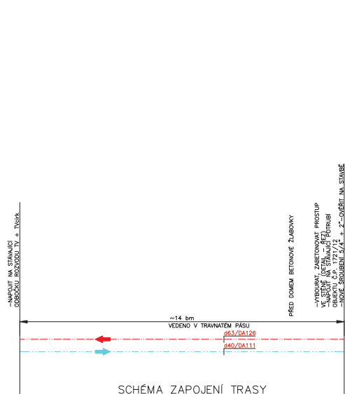
SCHÉMA ZAPOJENÍ TRASY
