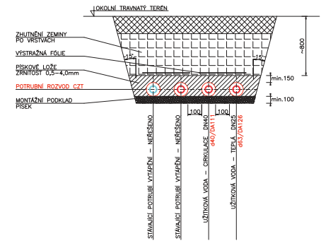
VZOROVÝ ŘEZ VÝKOPEM
